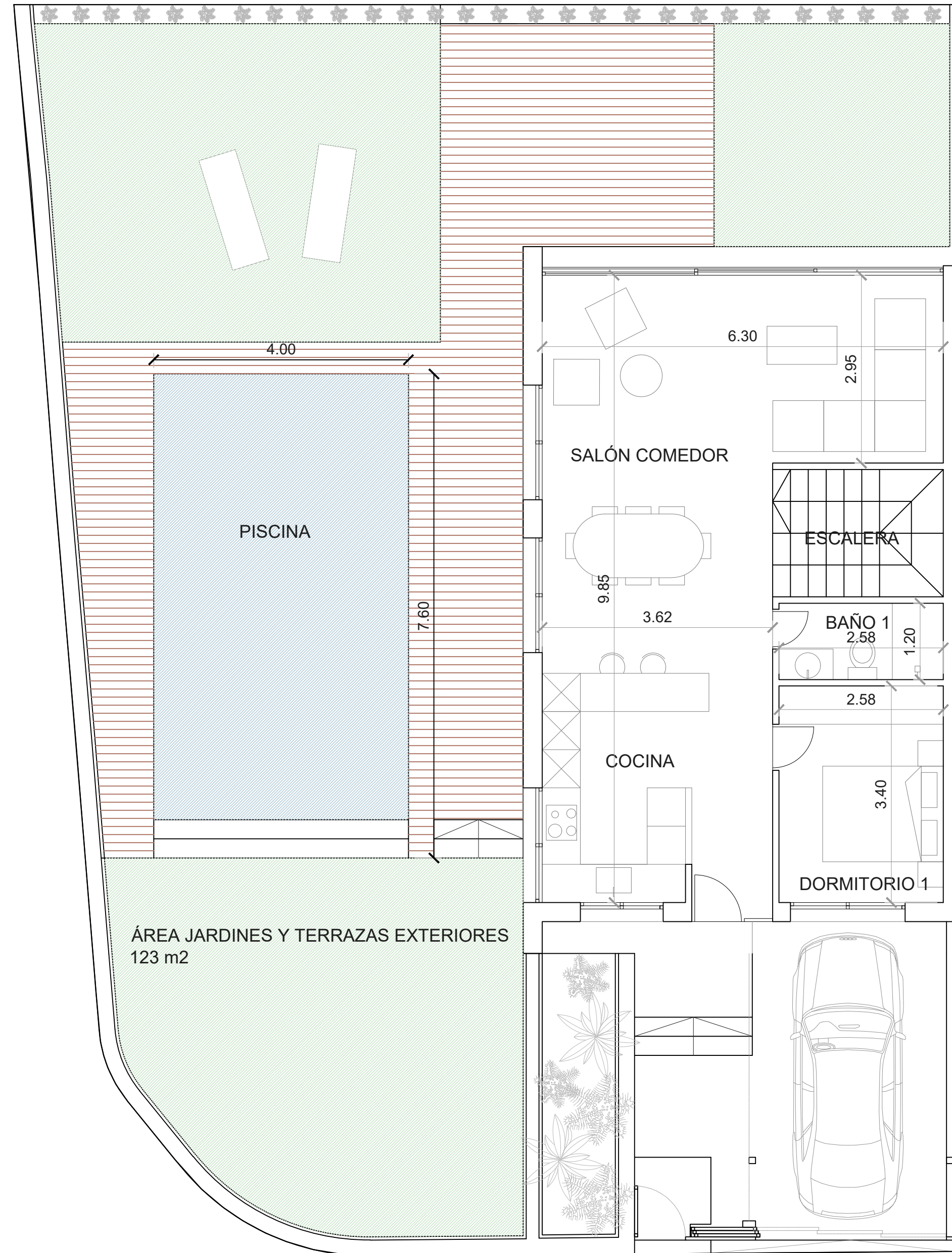
PLANTA BAJA
