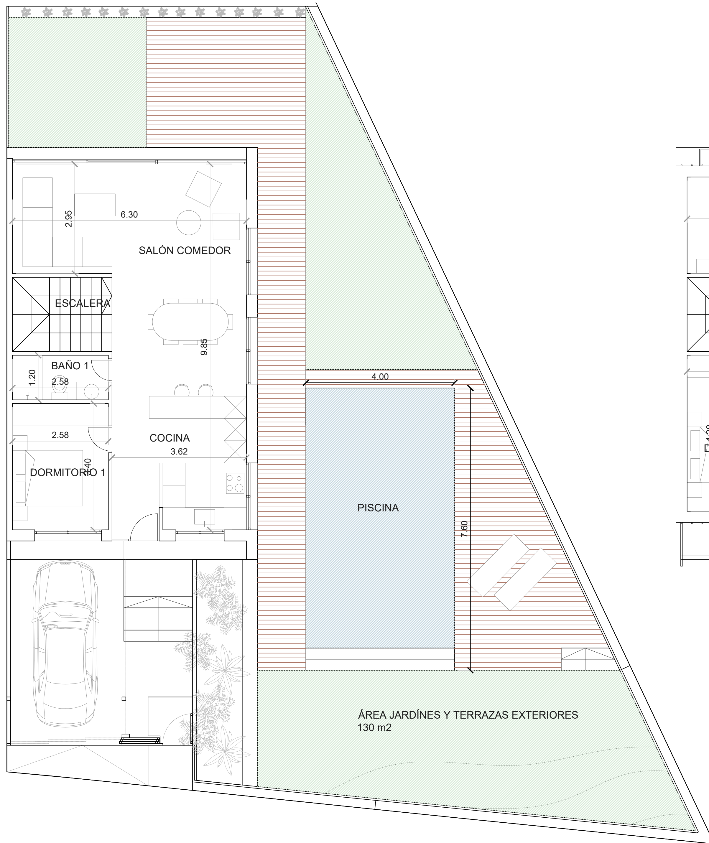
PLANTA BAJA
