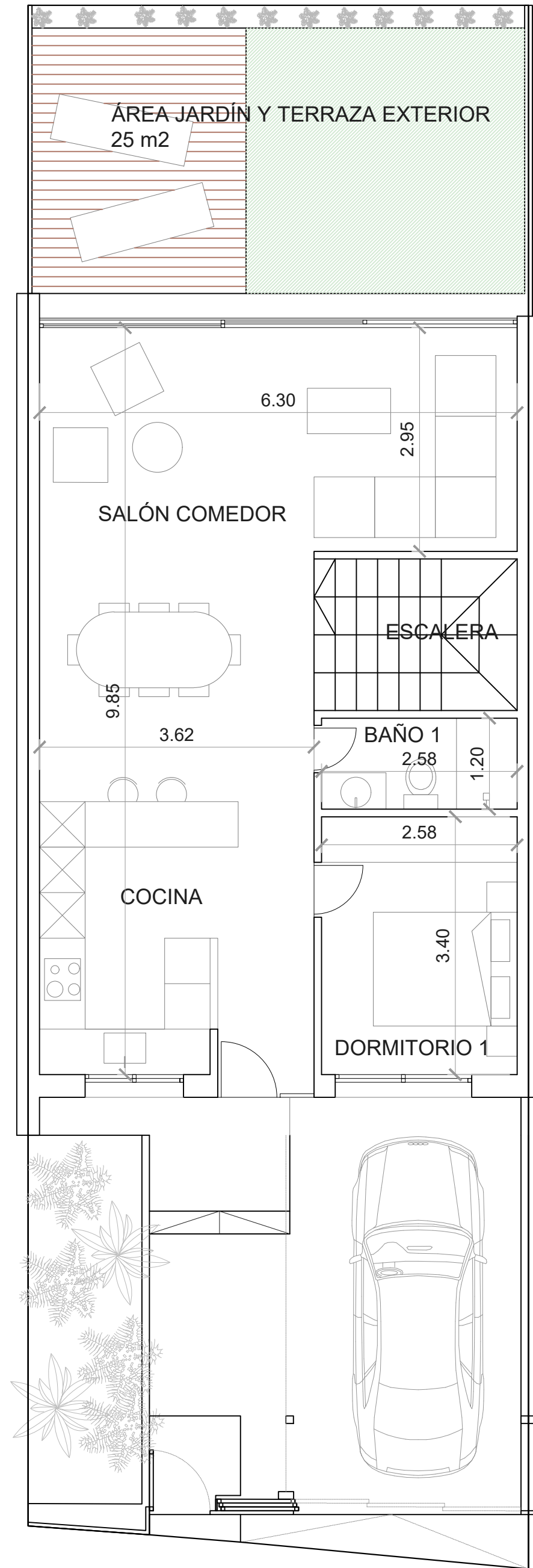
PLANTA BAJA
