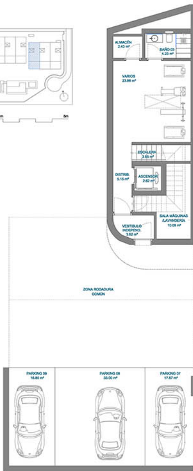
PLANTA SOTANO
