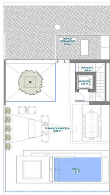
PLANTA SOLARIUM
