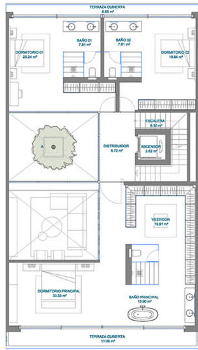
PLANTA PRIMERA
