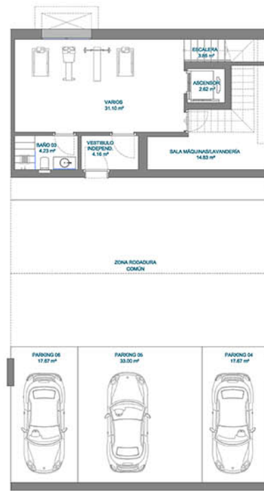
PLANTA SOTANO
