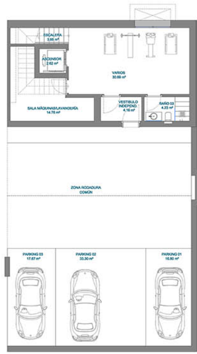
PLANTA SOTANA
