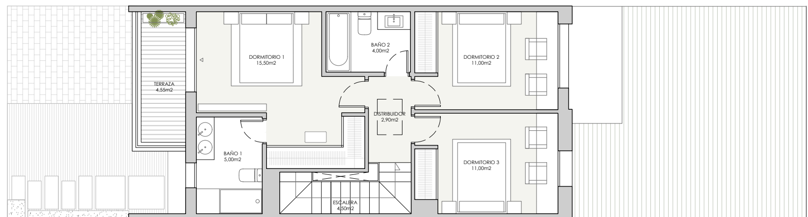
PLANTA PRIMERA
