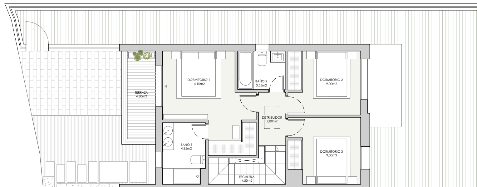
PLANTA PRIMERA
