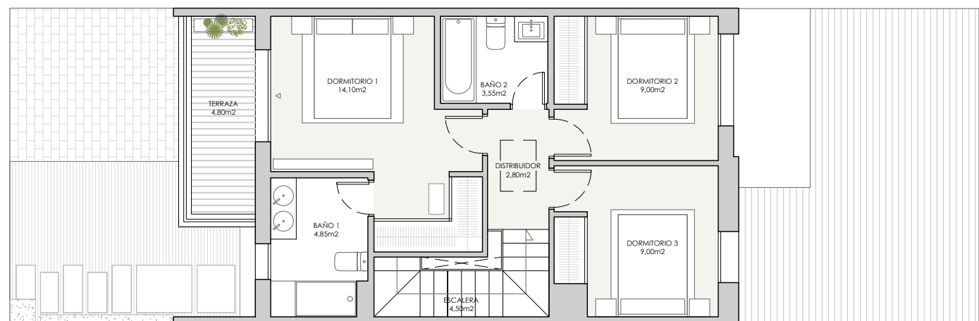
PLANTA PRIMERA
