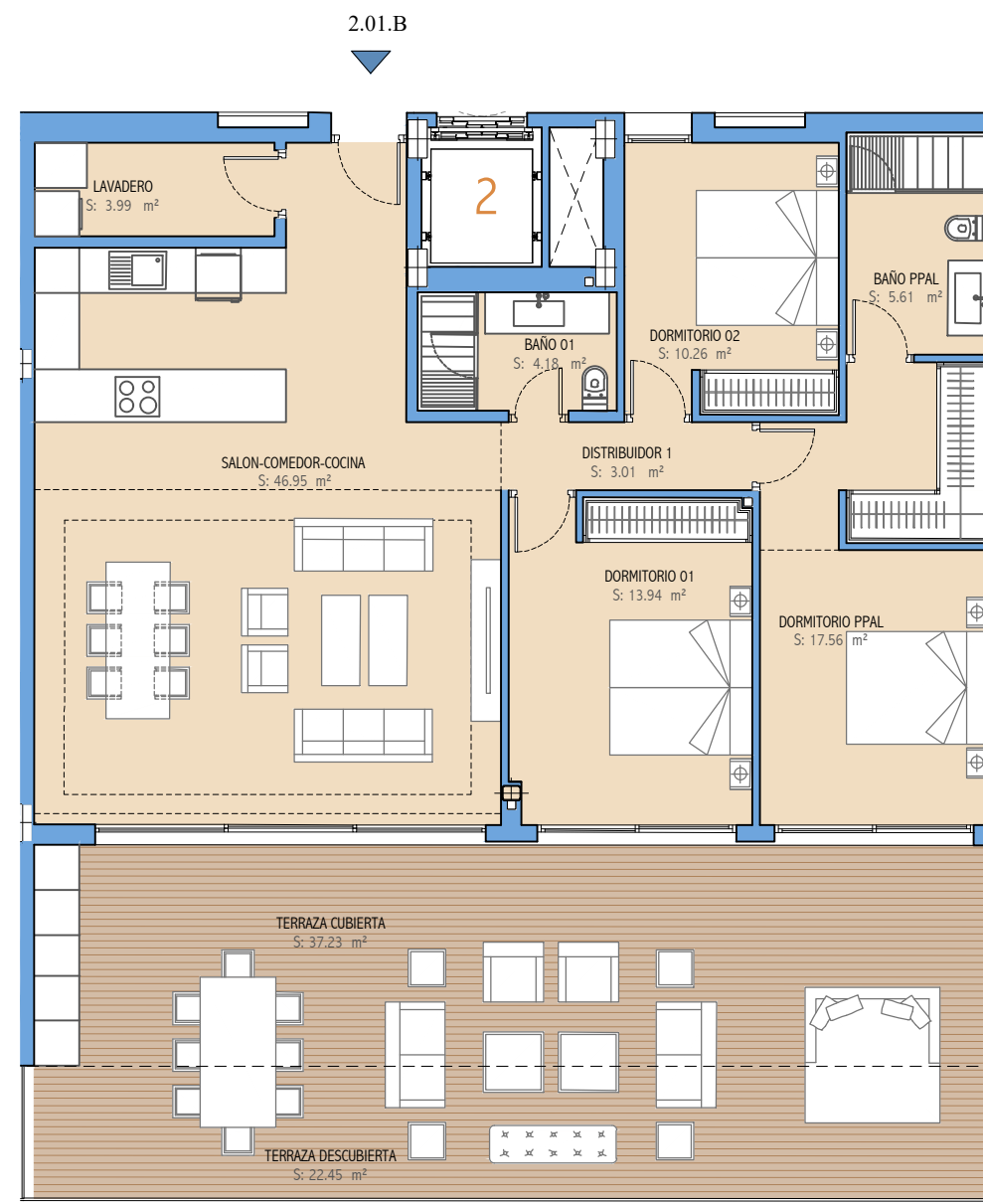
PLANTA PRIMERA
