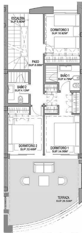
Planta Alta
