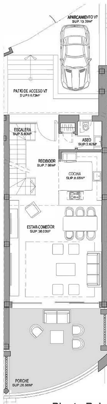
Planta Baja
