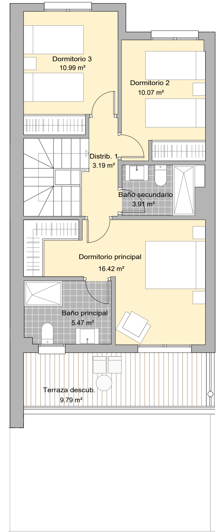
PLANTA PRIMERA
