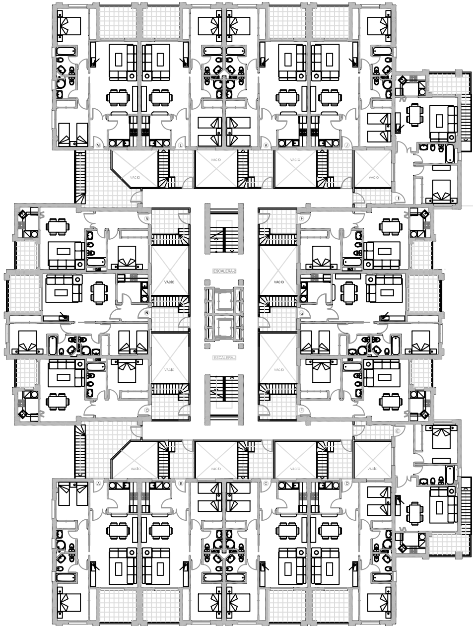
PLANTA TERCERA
