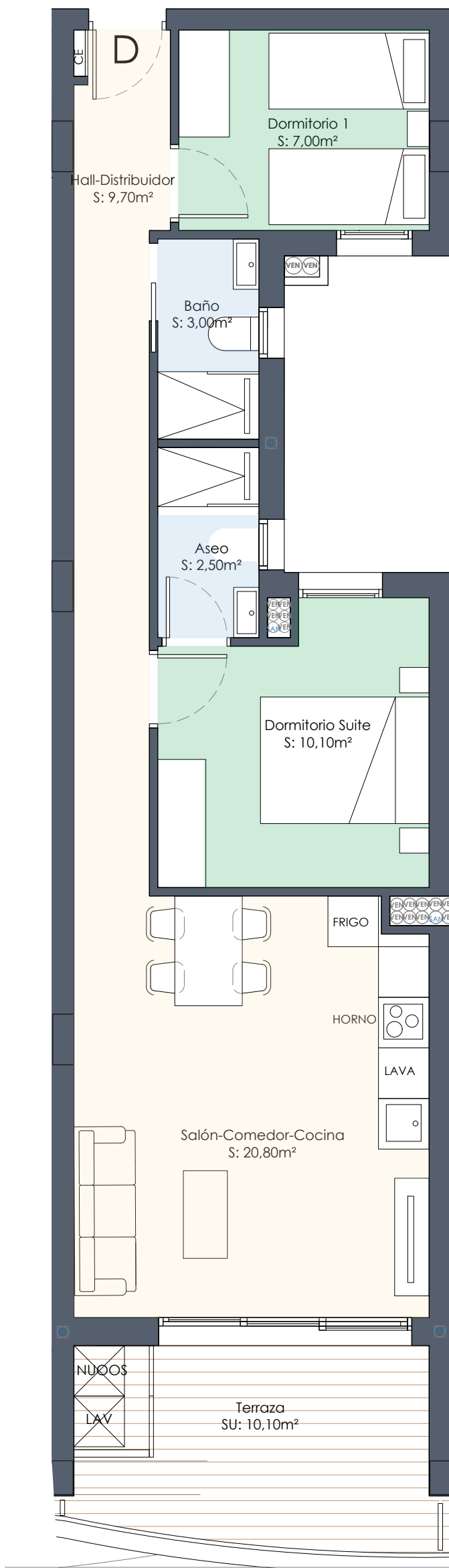
Planta Vivienda
