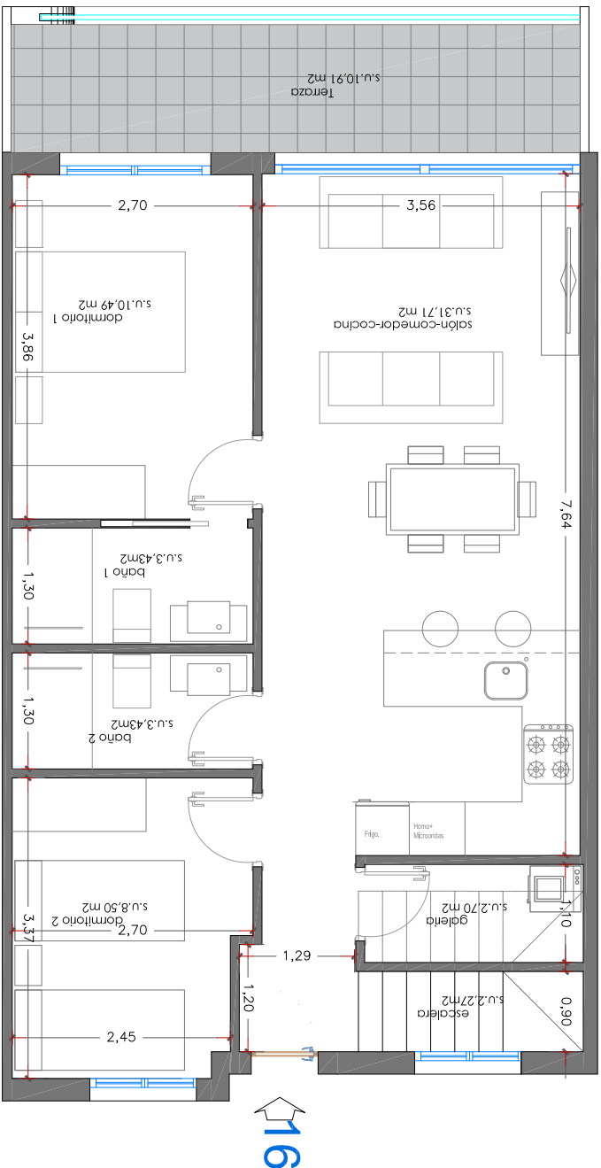
planta ático
