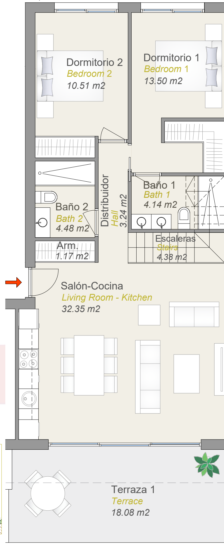
PLANTA PRINCIPAL
