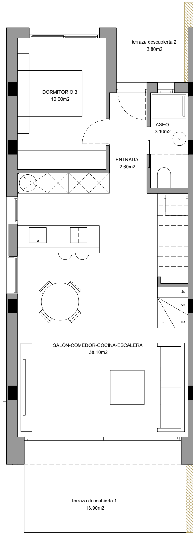
PLANTA BAJA - SUPERFICIES
