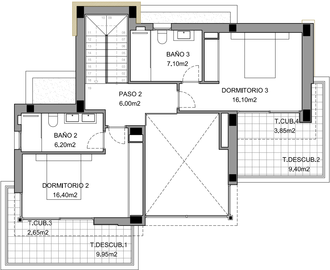
PLANTA ALTA - SUPERFICIES
